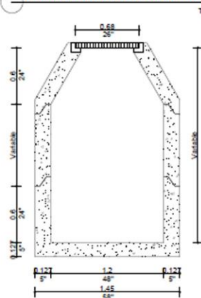
SECCIÓN DIMENSIONADA
