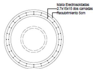
PLANTA ESTRUCTURAL
