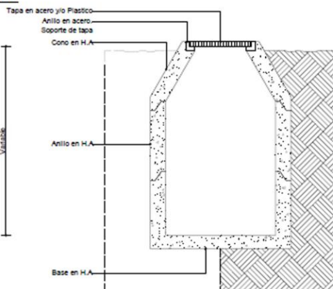
SECCIÓN DE MATERIALES
